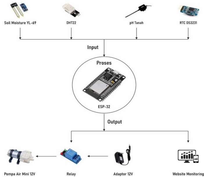
Gambar 2. Arsitektur Sistem Penyiraman Otomatis
