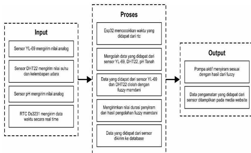
Gambar 1. Diagram Blok Sistem Penyiraman Otomatis
