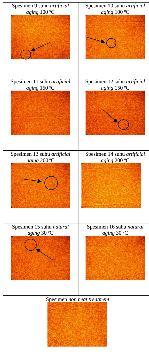
Gambar 6. Pengujian Struktur Mikro Solution Treatment 500 °C dengan Variasi Suhu pada Artificial Aging dan Natural Aging perbesaran 50x
