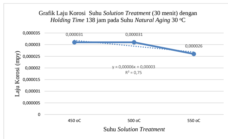
Gambar 4. Grafik Laju Korosi Terhadap Variasi Suhu Solution Treatment
